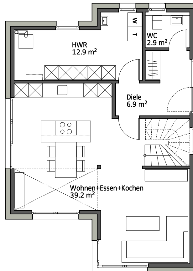
Erdgeschoss Variante B
