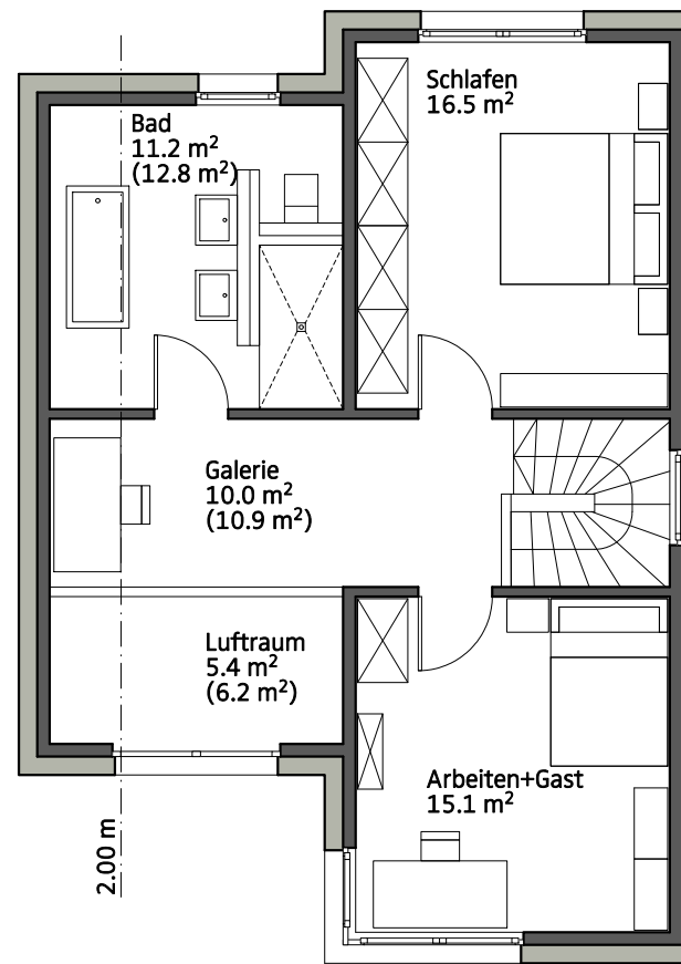
Dachgeschoss Variante B
