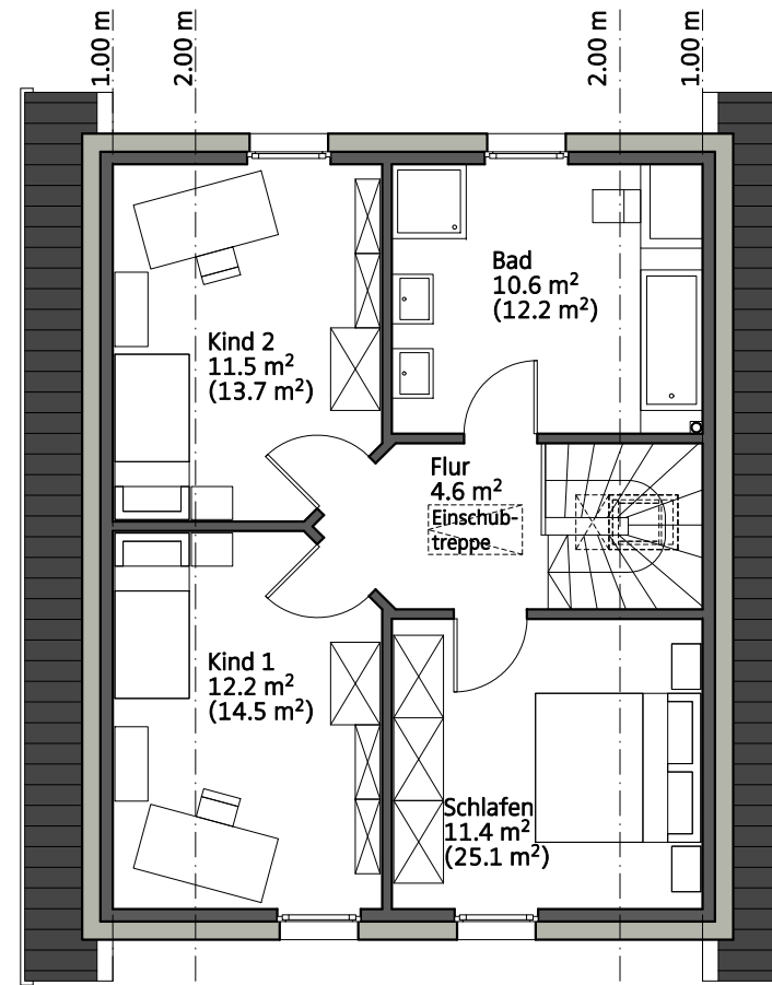
Dachgeschoss Variante B
