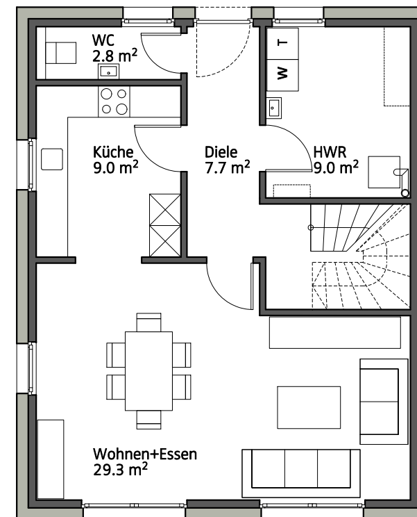
Erdgeschoss Variante B
